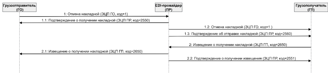
Рисунок 3.6 - Диаграмма последовательности отмены накладной грузоотправителем (один EDI-провайдер)
