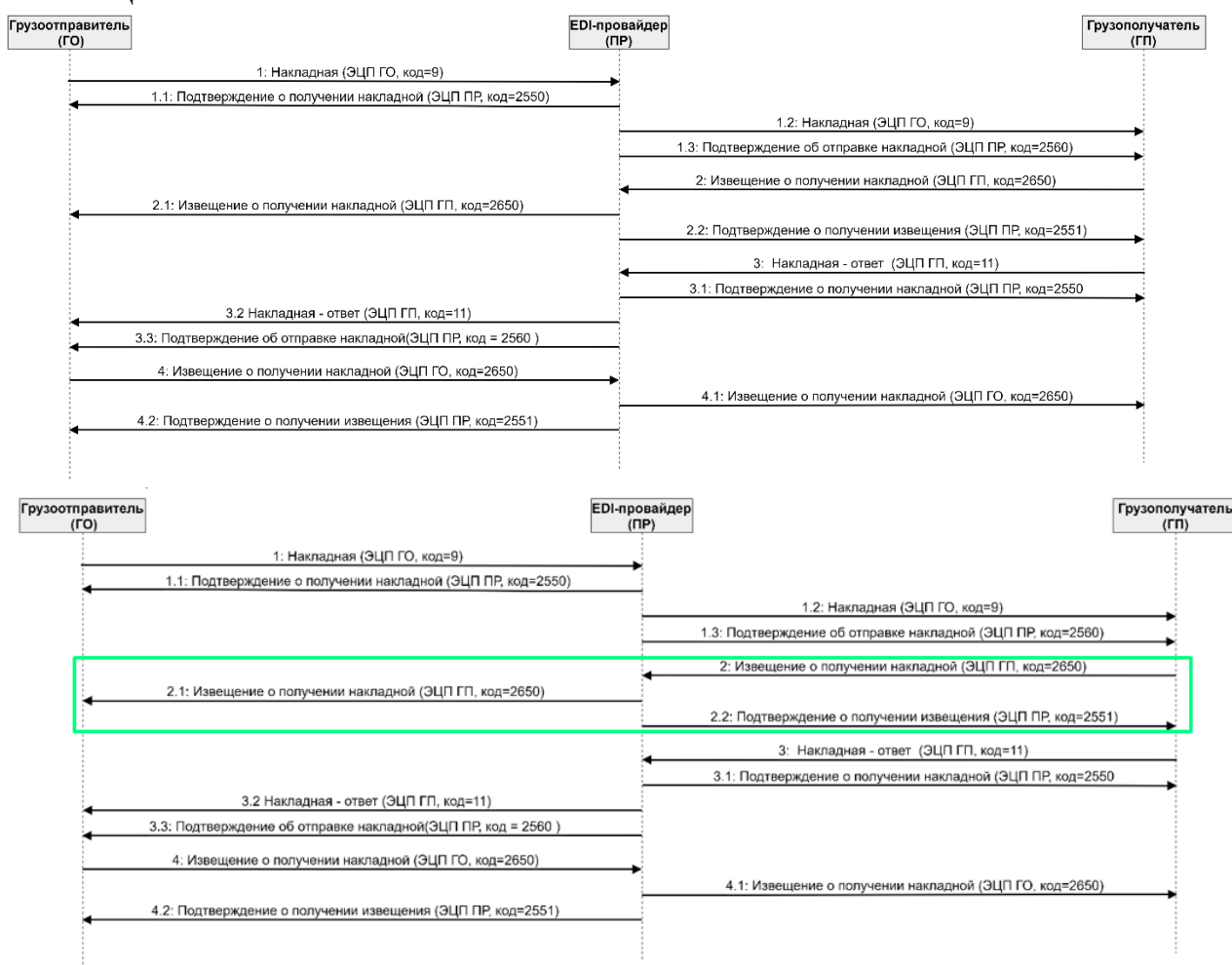
Рисунок 3.1 - Диаграмма последовательности передачи и подтверждения ЭТТН (один EDI-провайдер)
