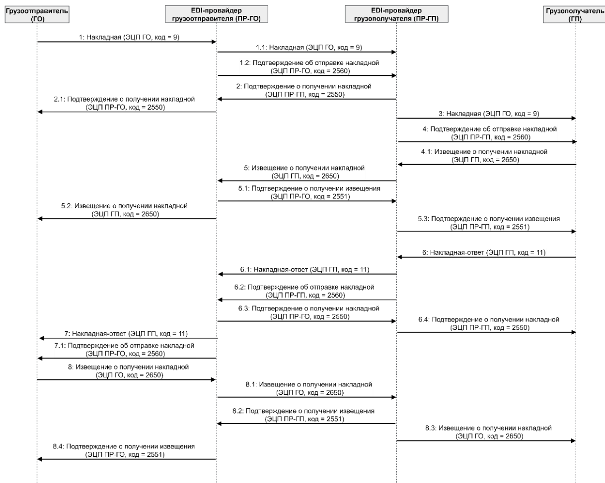
Рисунок 3.7 - Диаграмма последовательности передачи ЭТТН (два EDI-провайдера)
