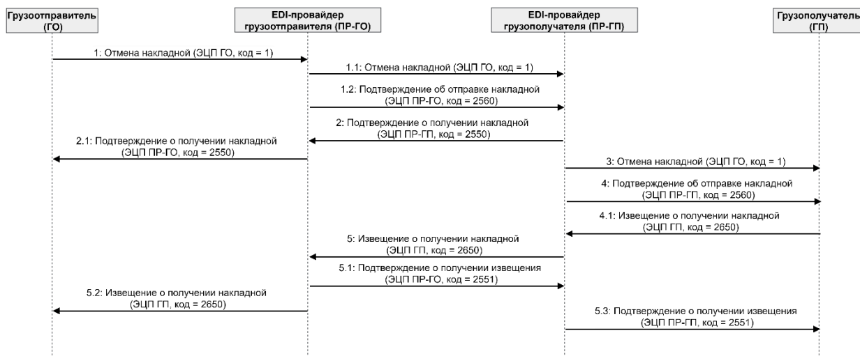
Рисунок 3.9 - Диаграмма последовательности отмены электронной накладной грузоотправителем (два EDI-провайдера)
