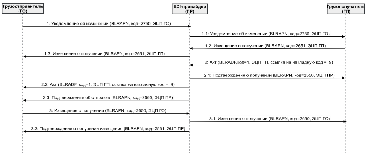
Рисунок 3.16 – Диаграмма последовательности изменения электронного акта приемки (один EDI-провайдер)
