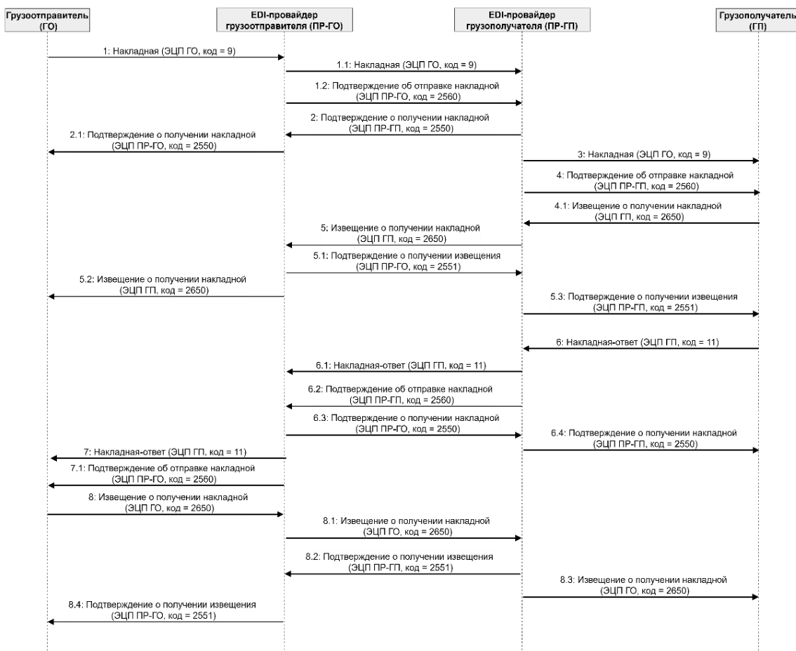
Рисунок 3.10 - Диаграмма последовательности передачи и подтверждения ЭТН (два EDI-провайдера)
